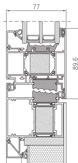
PRŮŘEZ DVEŘÍ TM 77N PRESTIGE S NADSVĚTLÍKEM
