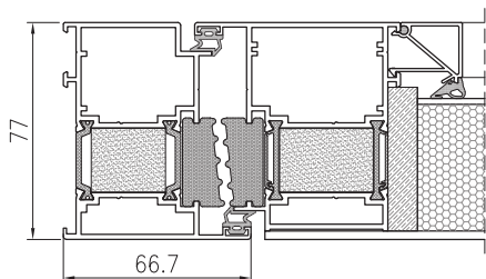
PRŮŘEZ DVEŘÍ TM 77N PRESTIGE
