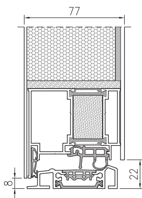
PRŮŘEZ DVEŘÍ TM 77N PRESTIGE
